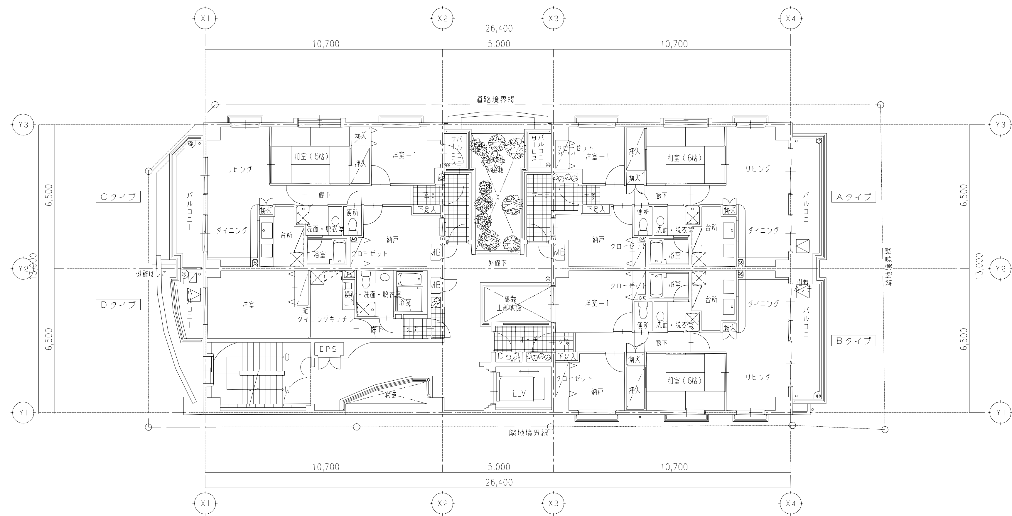
基準階 平面図
